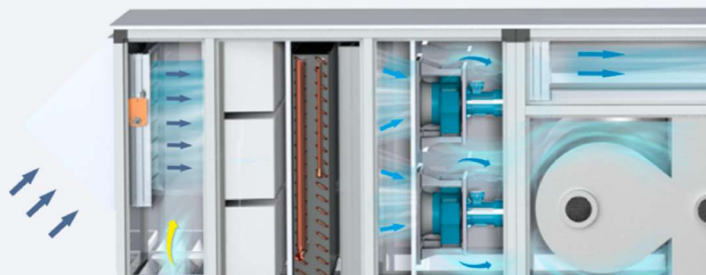
Приточно-вытяжные установки с рекуперацией (центральные кондиционеры)
